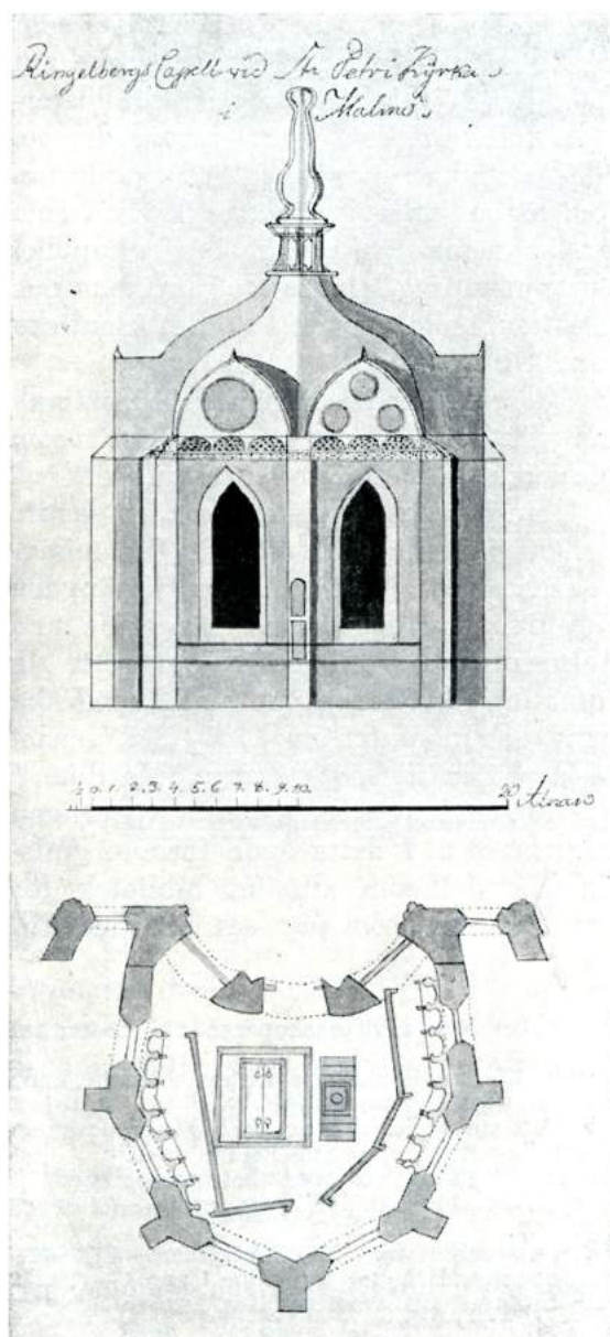
Fasad och planritning av Dringelbergska ka- pellet, uppgjord 1791 i samband med riv- ningsfrågan. (Efter original i Riksarki- vet.) Ringelbergska eller Munckekapellet var den gängse be- teckningen under 1700-talet
